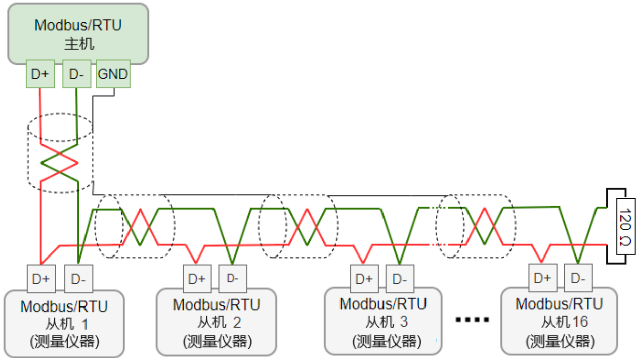
用 RS-485 分线器连接菊花链
