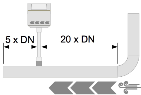
90° 拐角
