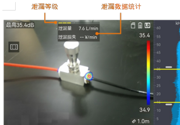
气体泄漏分析示意图
