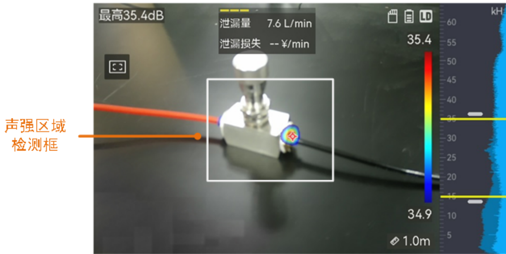
声强检测区域框
